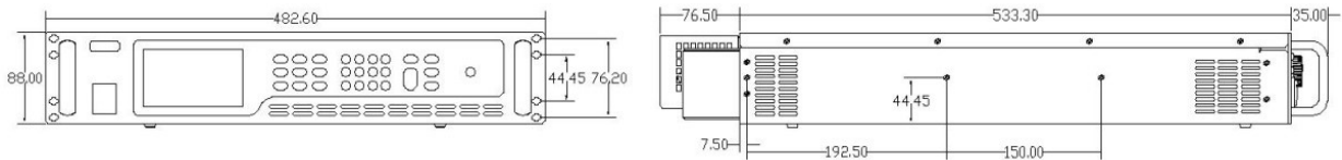
1. 6kW、2kW、3. 2kW机型尺寸图（10V、20V机型）：
