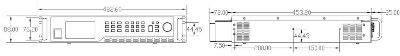
2kW、3. 2kW机型尺寸图（40V~1500V机型）：
