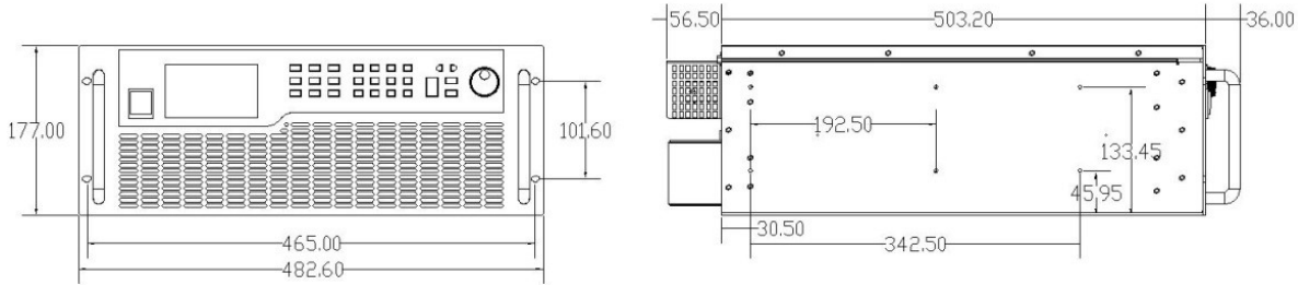
6. 5kW机型尺寸图（40V~1500V机型）：
