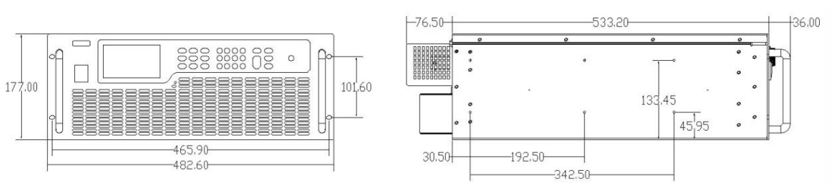
4. 8kW、6. 5kW机型尺寸图（10V、20V机型）：
